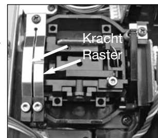
Uitgelichte veer voor gas links (mode 2+4)
