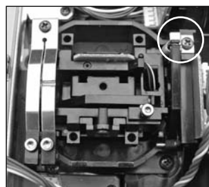
Uitgelichte terugstelveer voor gas rechts (mode 1+3)
