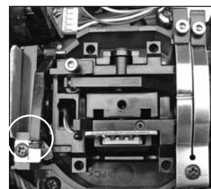
Uitgelichte veer voor gas links (mode 2+4)
